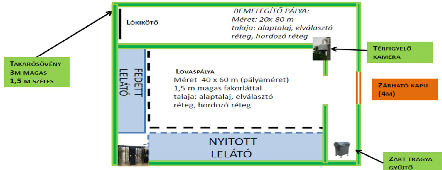
10. ábra Nyitott lovaspálya elvi vázlata (Saját tervezés)
