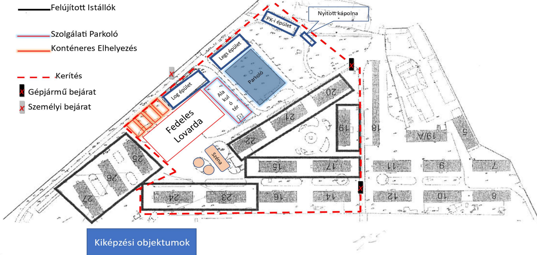
4. ábra Kincsem Park Huszárlaktanya- fejlesztési tervek 120 lóra
